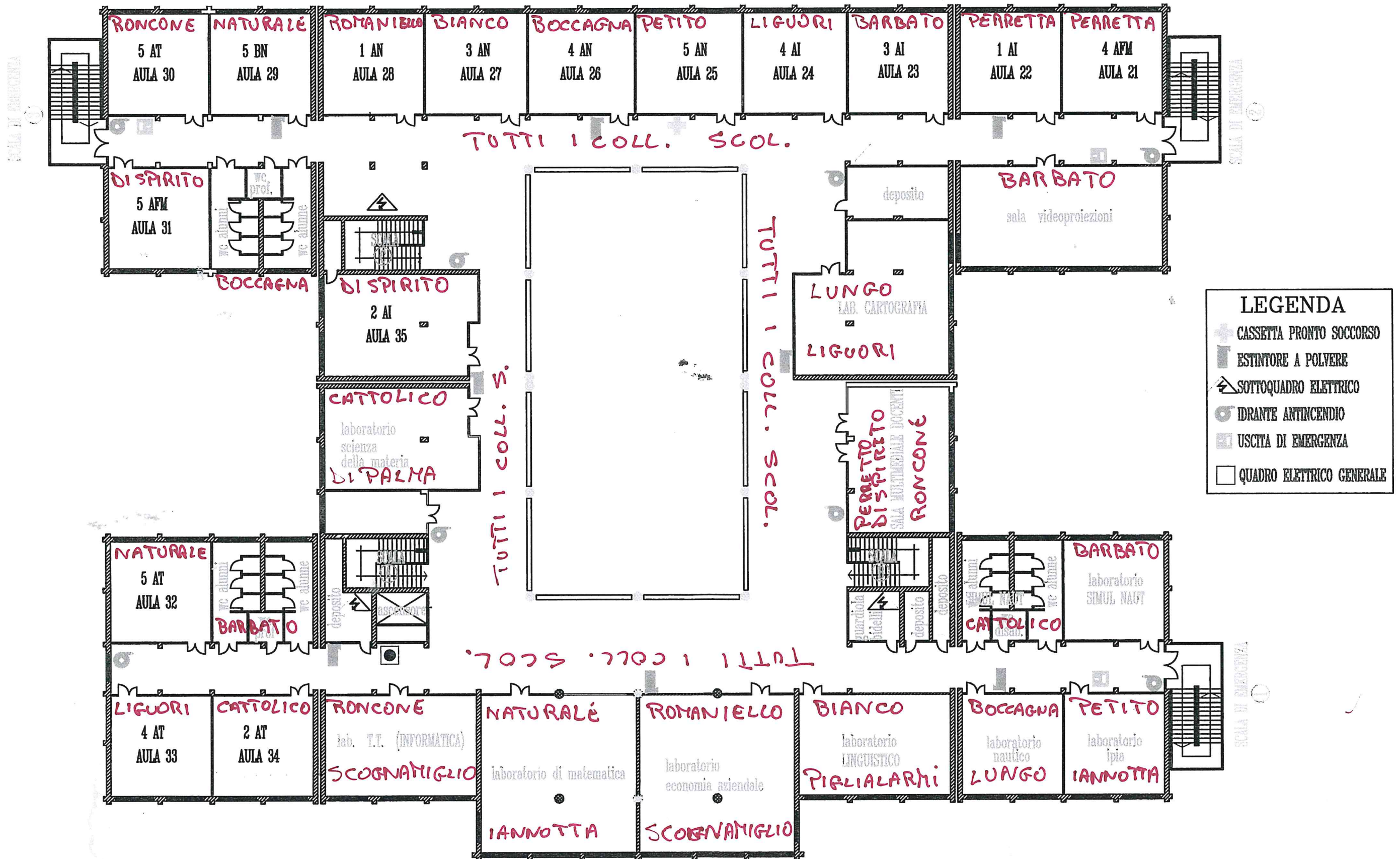
PIANTA PRIMO PIANO
